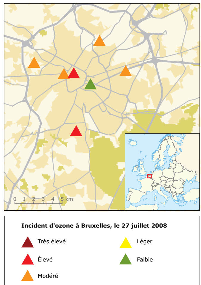
Fig. 1 / L'emplacement et les niveaux d'ozone aux stations de surveillance de la qualité de l'air à Bruxelles le dimanche 27 juillet 2008. Lorsque le relevé d'ozone dépasse les niveaux sains, un triangle rouge est affiché. Le gouvernement local doit alors en informer la population et proposer des mesures de précaution. Source : AEE, 2008.
